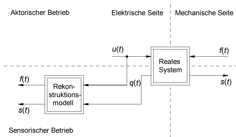
Bild 2: Piezoelektrischer Wandler als smarterer Aktor
