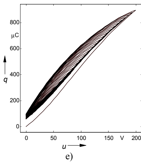
Bild 1: Gemessenes Übertragungsverhalten eines piezoelektrischen Wandlers bei elektrischer Großsignalaussteuerung (Erläuterung im Text).
